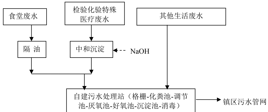
图 4-1 本项目污水处理工艺流程图
