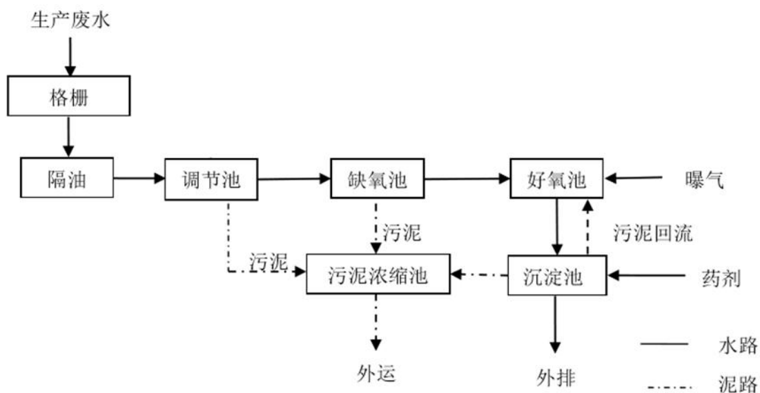
图 4.2-1 一体化污水处理设备工艺流程图
