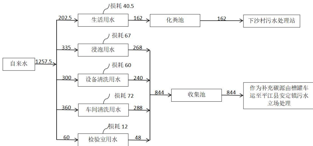
图 2-1 近期水平衡图 (单位: \text{m}^3/\text{a} )
