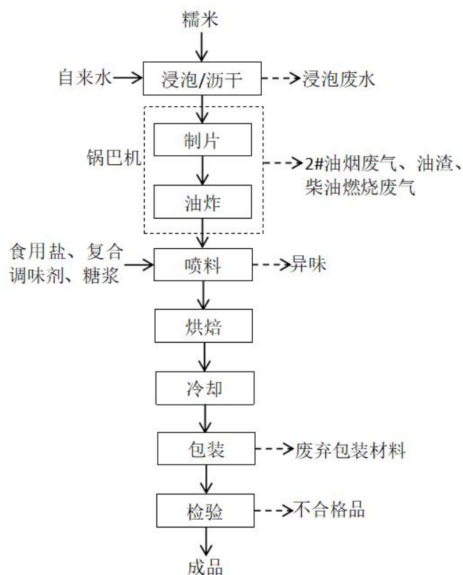
图2-3 炒米锅巴生产工艺流程图及产污环节图
