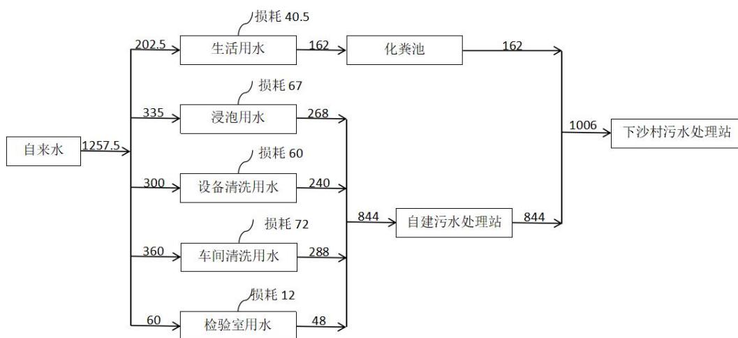
图 2-2 远期水平衡图 (单位: m^3/a )
