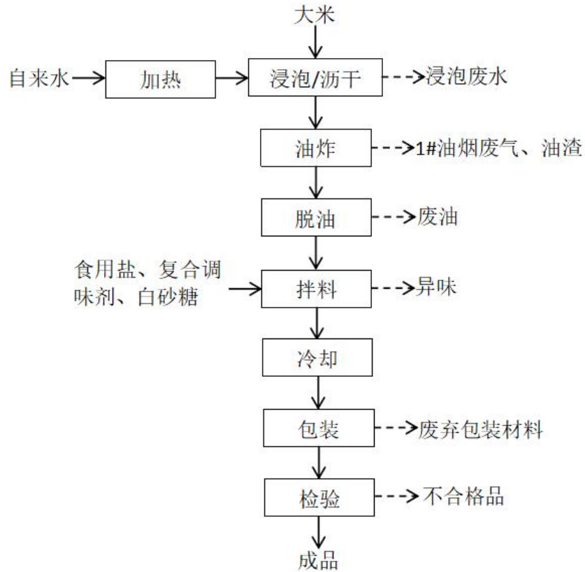
图2-2 炒米生产工艺流程及产污环节图
