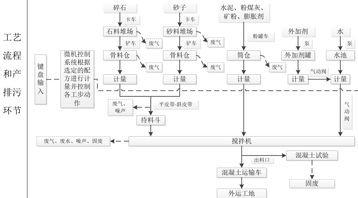
图 2.9-1 运营期项目工艺流程及产排污环节示意图
