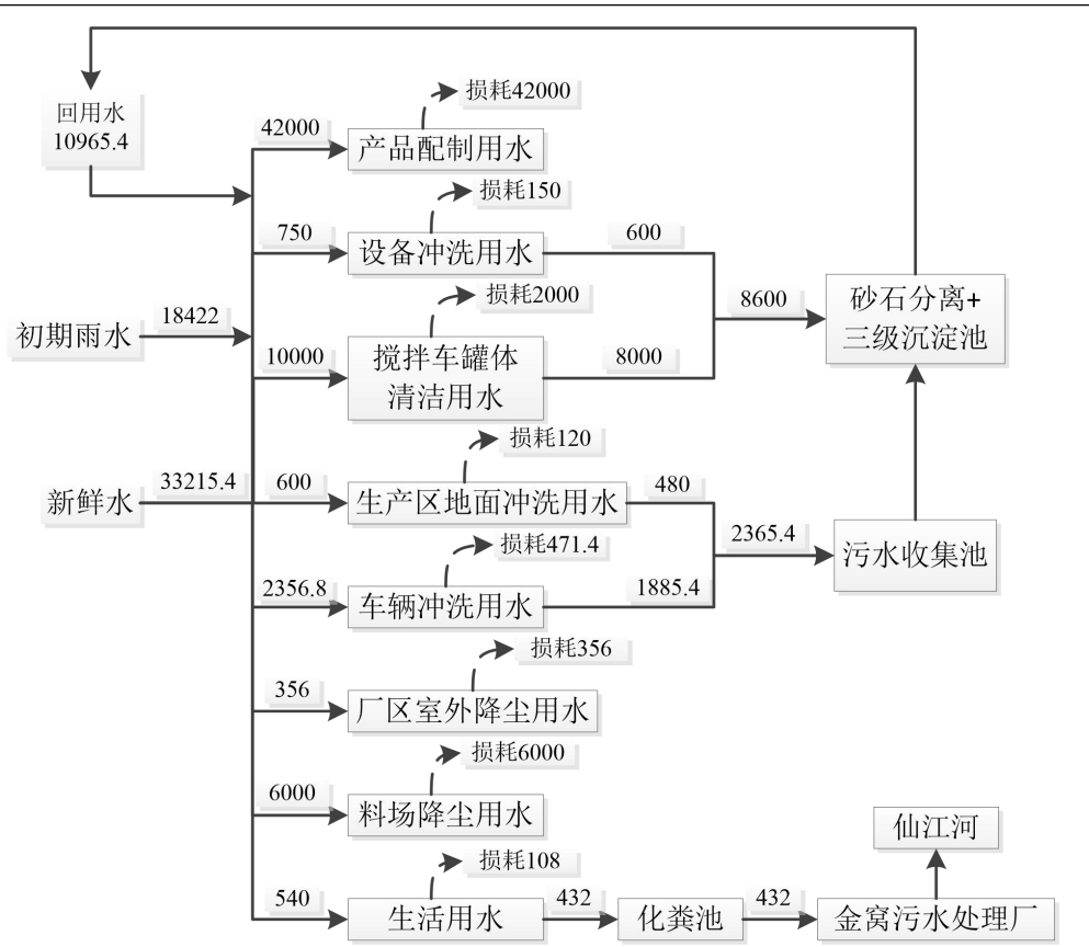
图 2.6-1 项目水平衡图 (单位: m^3/a )
